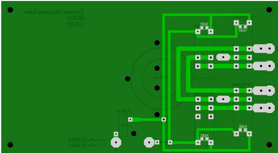
DK2CH-Balun-V2.02-BOT
