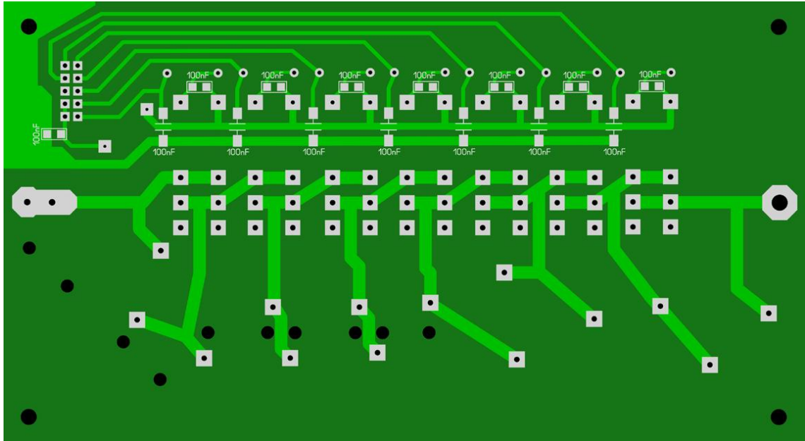
DK2CH-Spulen-Platine-2-BOT
