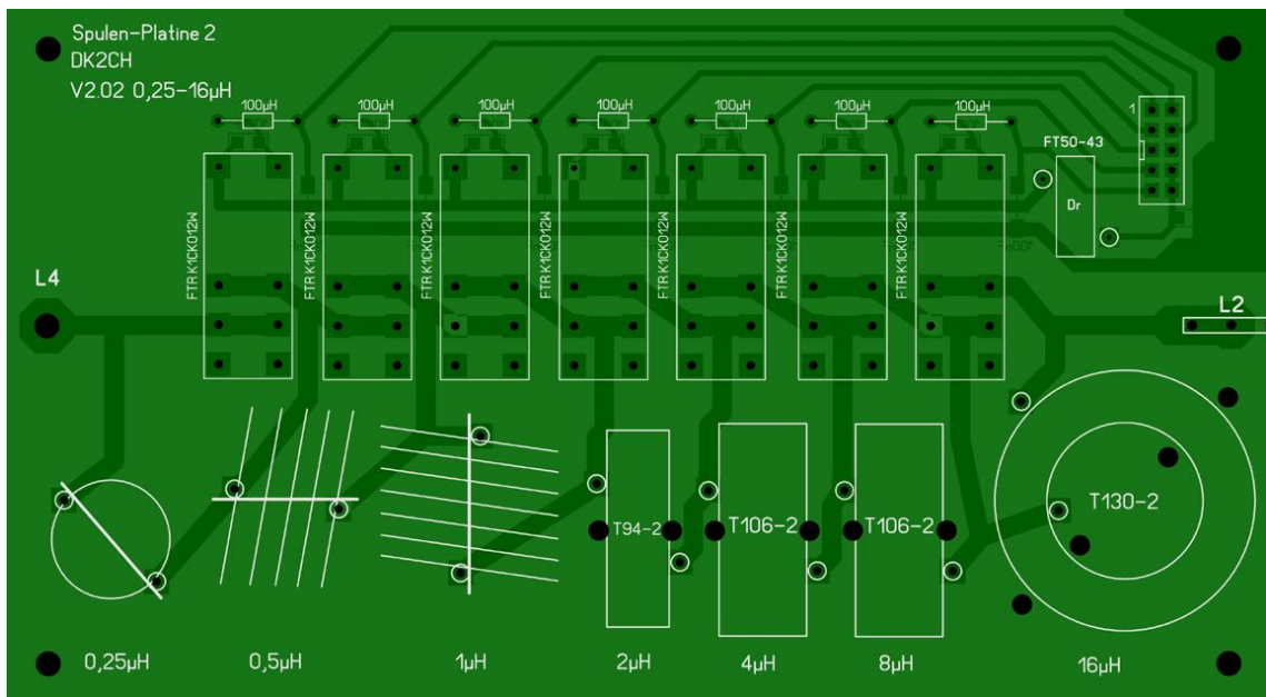
DK2CH-Spulen-Platine-2-TOP
